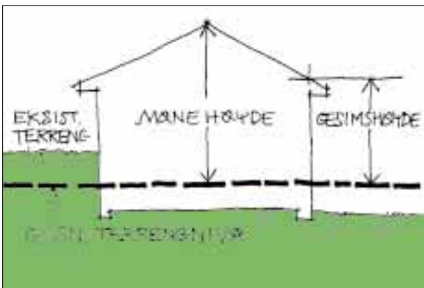
Figur 91 - Gesimshøyde måles til skjæringspunktet mellom veggliv og takflate, dvs oppå takflaten. Der brystning eller parapet er høyere enn 0,3 m, måles høyden til overkant av brystning. Høyden skal måles fra gjennomsnittlig terrengnivå rundt bygningen.
