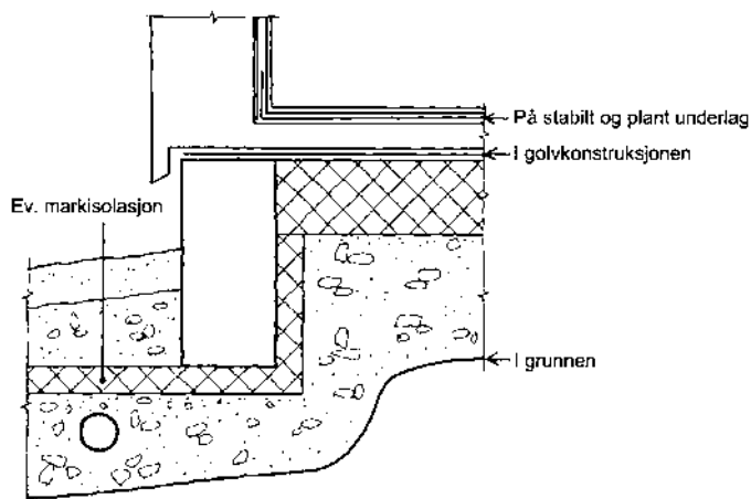
§ 8-33 fig. 3 Prinsippskisse av alternative plasseringer av radonsperre
