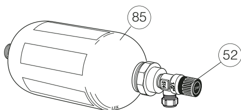
Nivåkärl med säkerhetsventil
