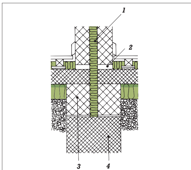
Figur C37 Overgang mellom tung skillevegg og gulv på grunn
