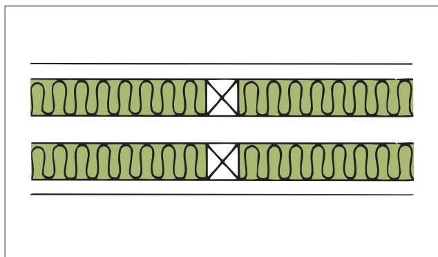
Figur C2 Isolert vegg med Rockwool R_w = 57 dB
