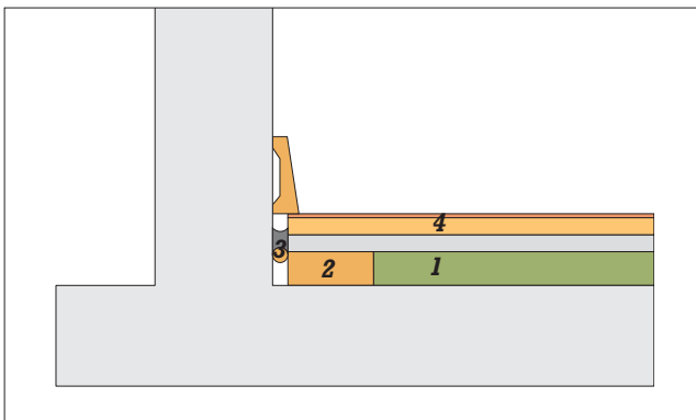
Figur D3 Kantunderstøttelse
