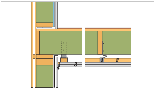
Figur D4 Overgang mot yttervegg av tre
