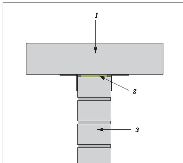
Figur C40 Overgang mellom tung skillevegg og etasjeskiller med branntetting
