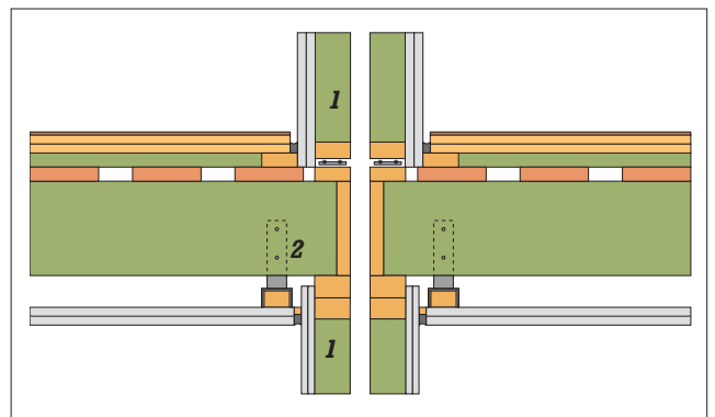
Figur D6 Overgang mot dobbel lydvegg
