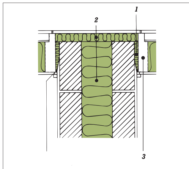
Figur C38 Overgang mellom tung skillevegg og lett yttervegg
