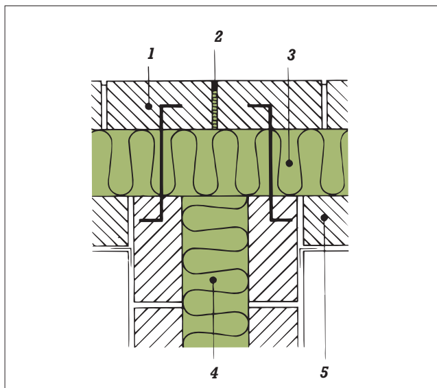
Figur C39 Overgang mellom tung skillevegg og tung yttervegg
