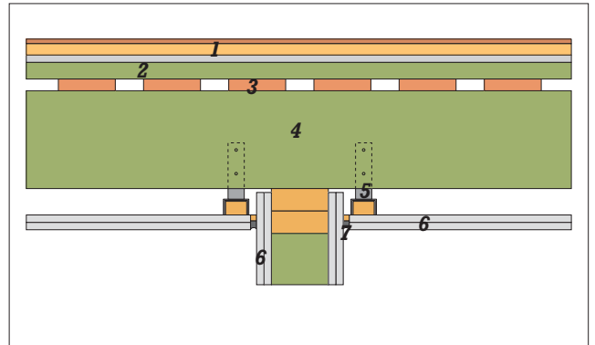
Figur D5 Overgang mot lett bærevegg
