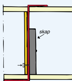
Fig. 3 Vertikal rørføring
