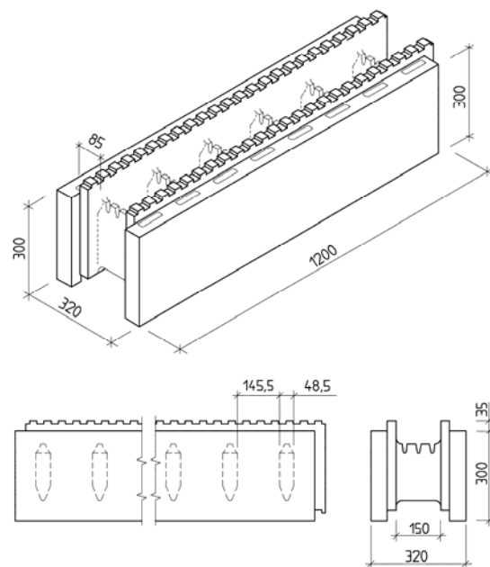
Fig. 1 Kub standardblokk. Mål i mm
