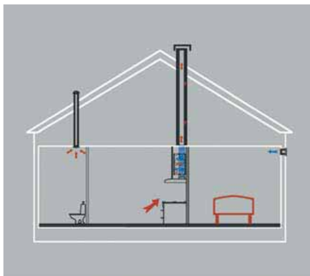
Enebolig – normalventilasjon
